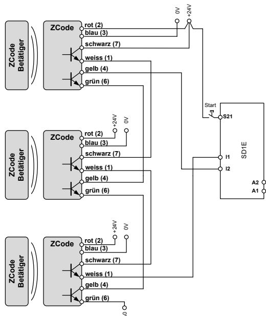
Abb. 8: Anschluss von bis zu 3 ZCodes in Reihe an ein ZANDER MINOS SD1E
