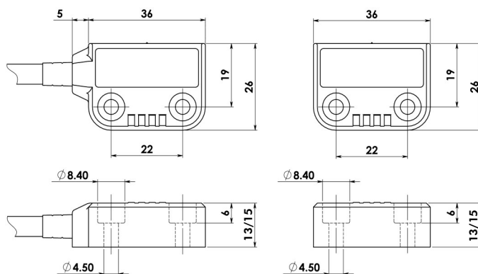
Schalter ZCode-TC / -TCE (Kabel rechts, Höhenmaß 13 mm bei TC und 15 mm bei TCE)
